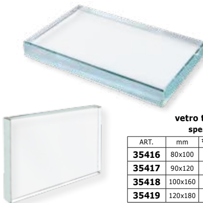
vetro trasparente spessore 19 mm
